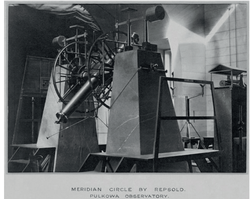
Меридианный круг. Обсерватория Пулково
